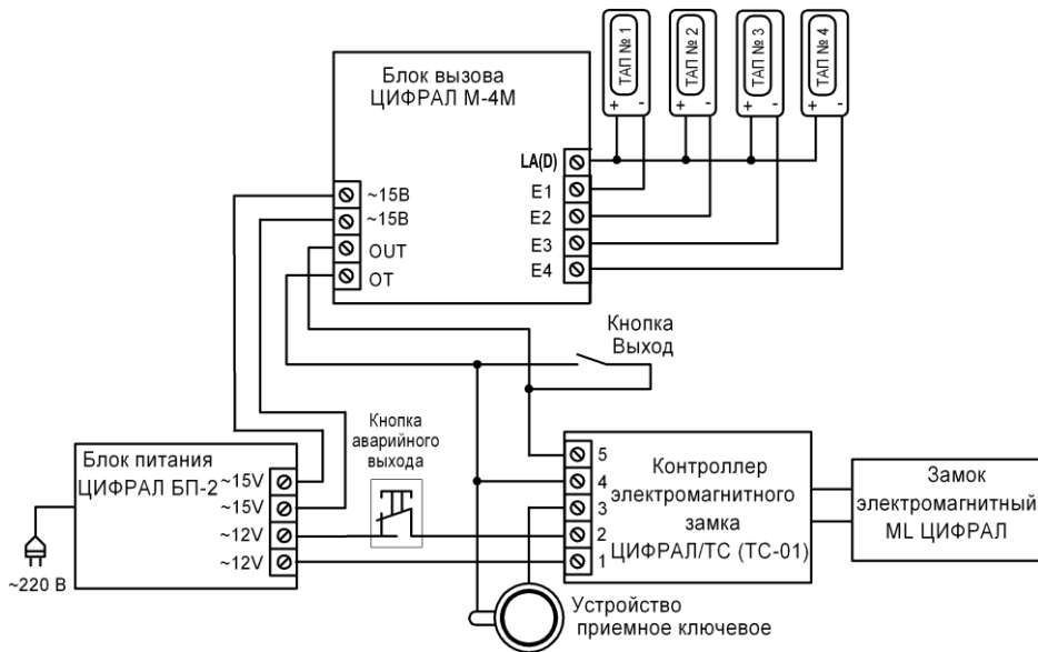
Рисунок Б.2 Схема подключения домофона ЦИФРАЛ М-4М
