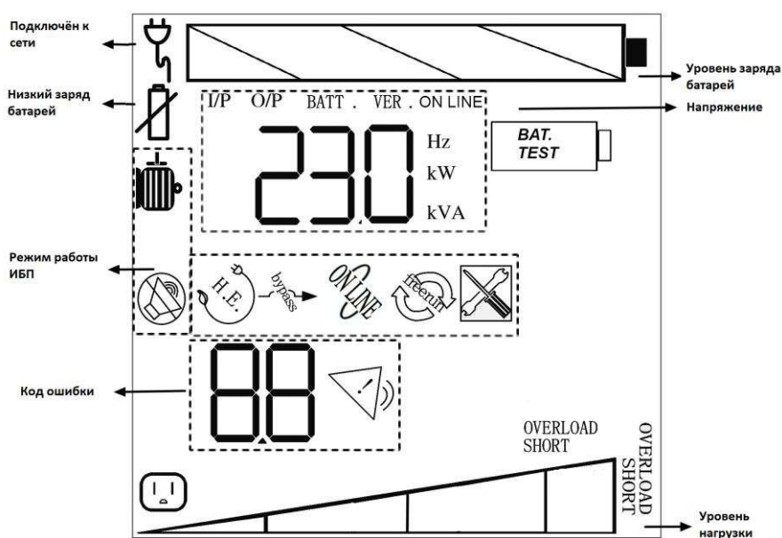
Рис. 7. ЖК-дисплей
