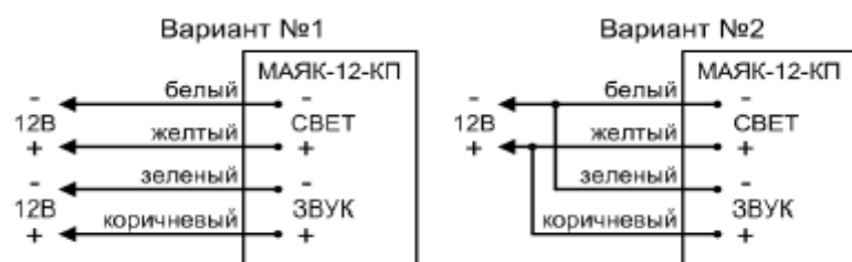
Рис.1 Схема подключения.
