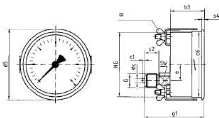
Эксцентрично-осевое исполнение со скобой - ТэСк
