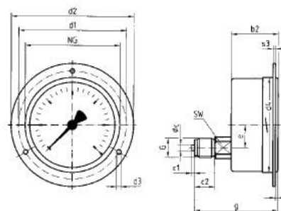
Эксцентрично-осевое исполнение с фланцем передним - ТэФп
