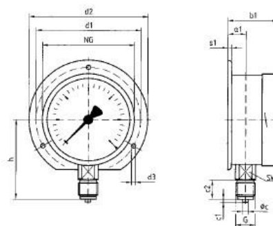
Радиальное исполнение с фланцем задним - РФз
