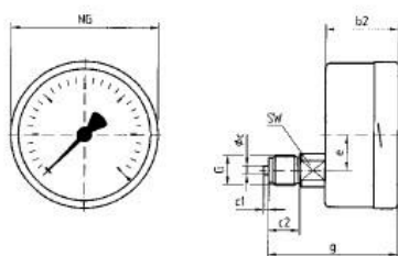
Эксцентрично-осевое исполнение - Тэ
