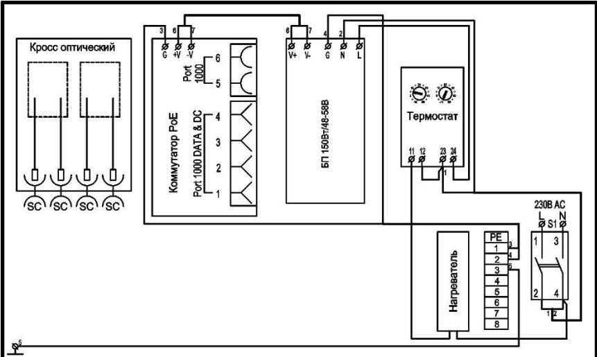
Рисунок 2 – Схема электрическая принципиальная
