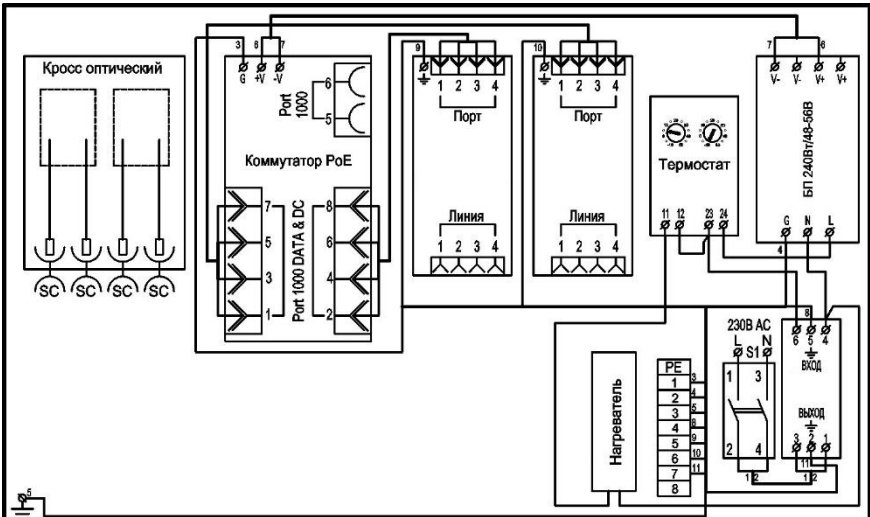
Рисунок 2 – Схема электрическая принципиальная
