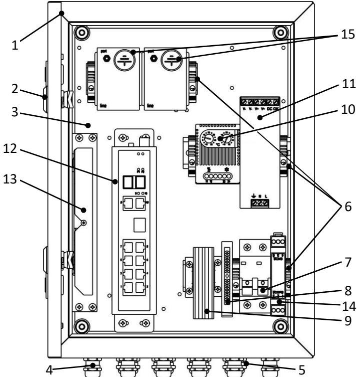
Рисунок 1 – Устройство шкафа
