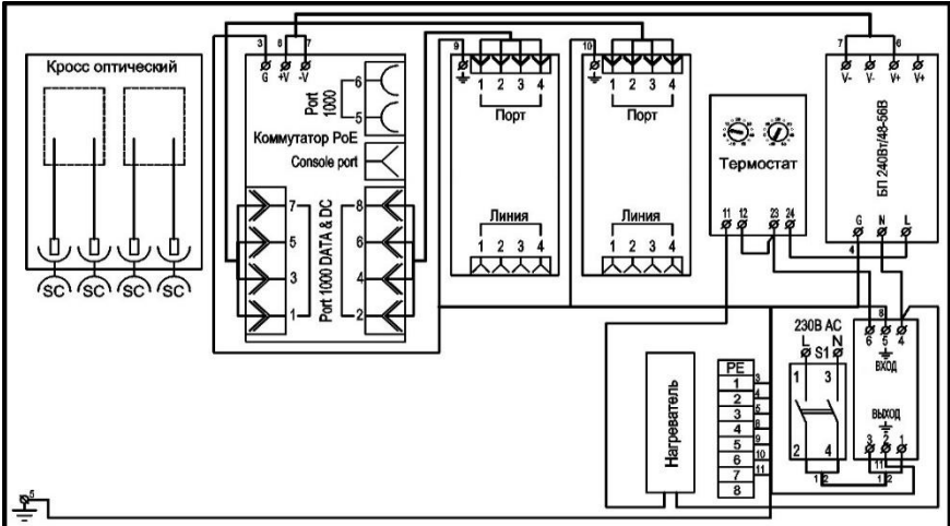
Рисунок 2 – Схема электрическая принципиальная
