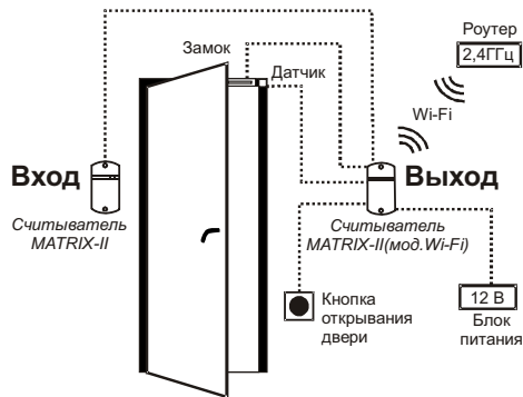
Рис.2 Схема подключения MATRIX-II (мод. Wi-Fi).
