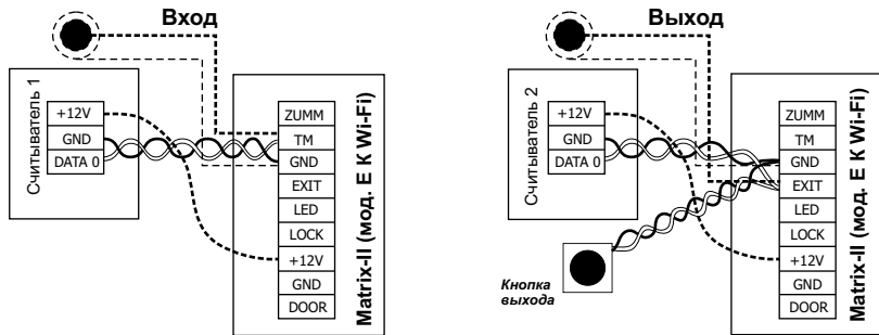
Рис.4 Подключение внешних считывателей по протоколу iButton
