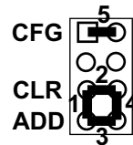
Рис.7 Перемычка
