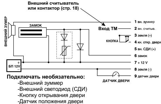
Рис. 5 Подключение внешних устройств
