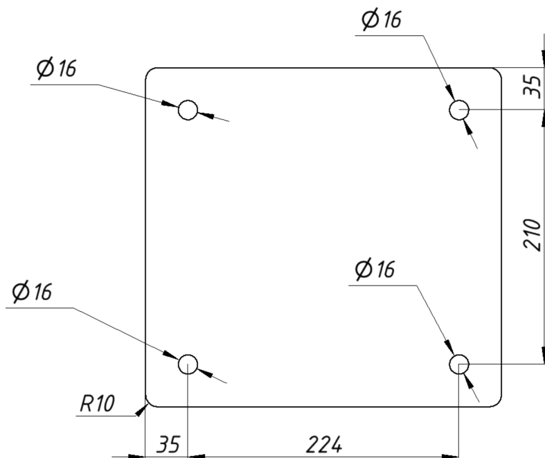
Рисунок 6.4.2. Монтажное основание.
