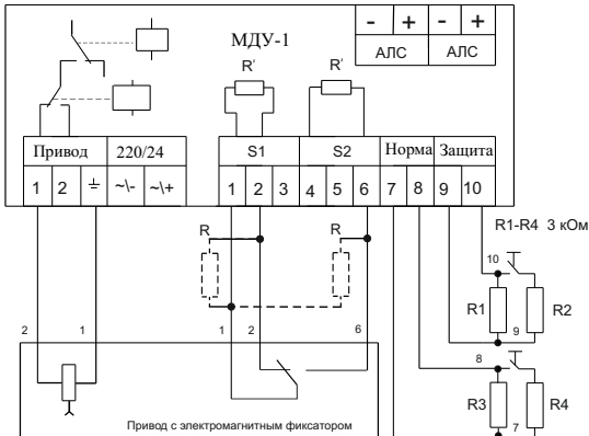
Рисунок 4 – Вариант подключения привода с электромагнитным фиксатором
