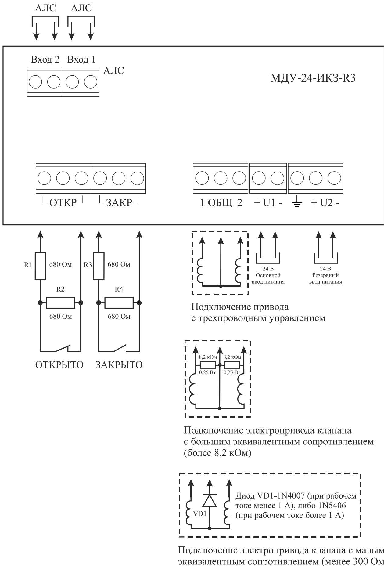
Рисунок 4.5 – Подключение реверсивного привода с концевыми выключателями с номинальным напряжением 24 В
