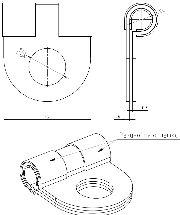
Рисунок 1. Чертёж МЭТ-04-02
