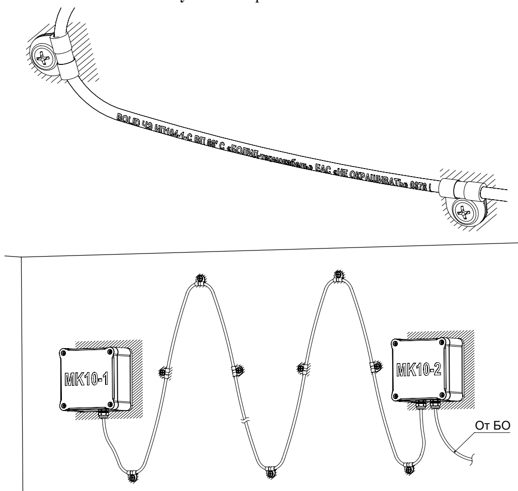
Рисунок 2. Пример размещения МЭТ-04-02
