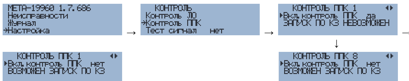
Рисунок 8. Включение / отключение контроля по шлейфам ПС.
