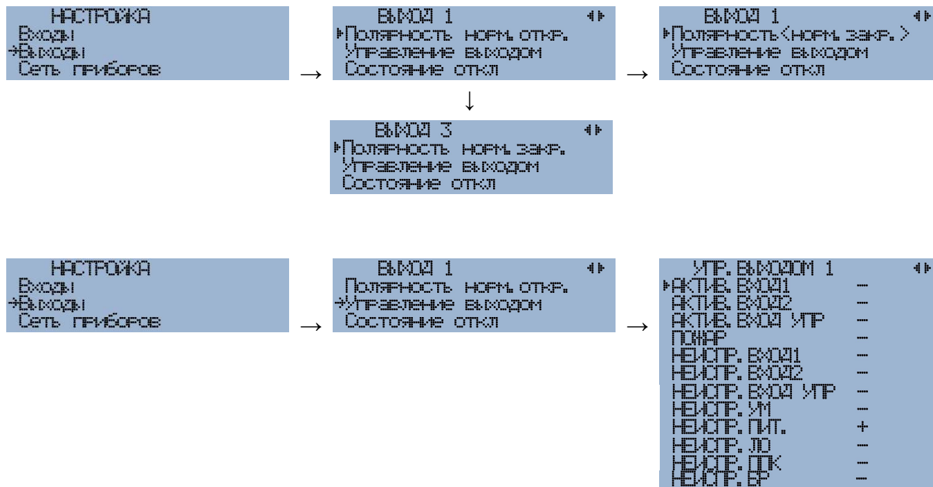
Рисунок 13. Настройка Выход 1, Выход 2, Выход 3.
