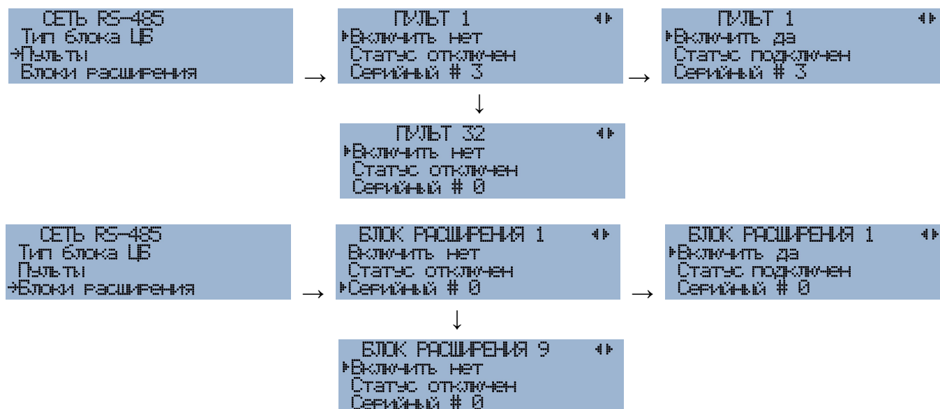
Рисунок 7. Настройка пультов и блоков расширения.
