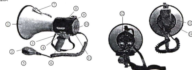
Рисунок. Конструкция ЭМ.
