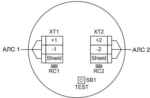
Рисунок Б.1 - Схема внешних подключений
