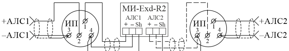
Рисунок Б.5 - Схема подключения МИ-EXD-R2 в АЛС кольцевого типа
