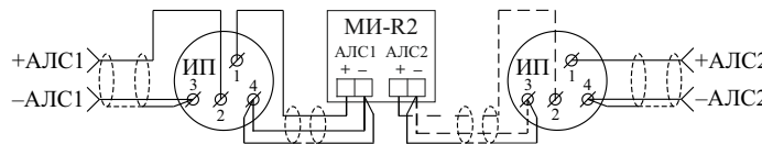
Рисунок 8 – АЛС кольцевого типа
