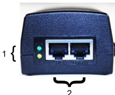
Рис. 1. Инжектор Midspan-1/190A , Midspan-1/300A Midspan-1/300G , вид спереди
