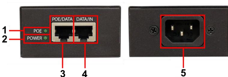
Рис. 2 Midspan-1/902G, разъемы на передней и задней панелях
