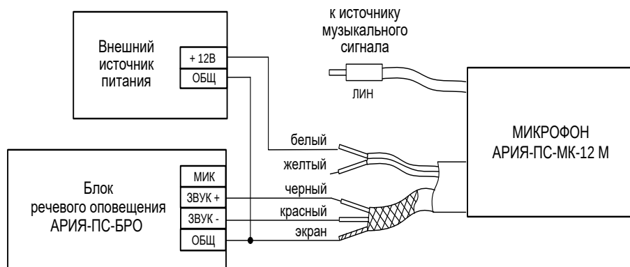
Рис.2. Схема соединений при подключении микрофона с минимальным приоритетом.
