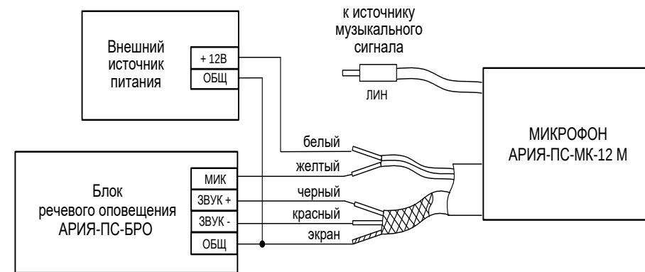
Рис.1. Схема соединений при подключении микрофона с максимальным приоритетом.
