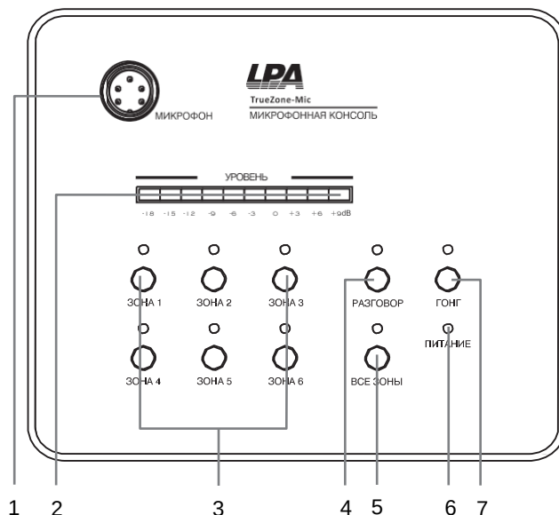
Рис. 2.1. LPA-TrueZone-MIC (передняя панель)
