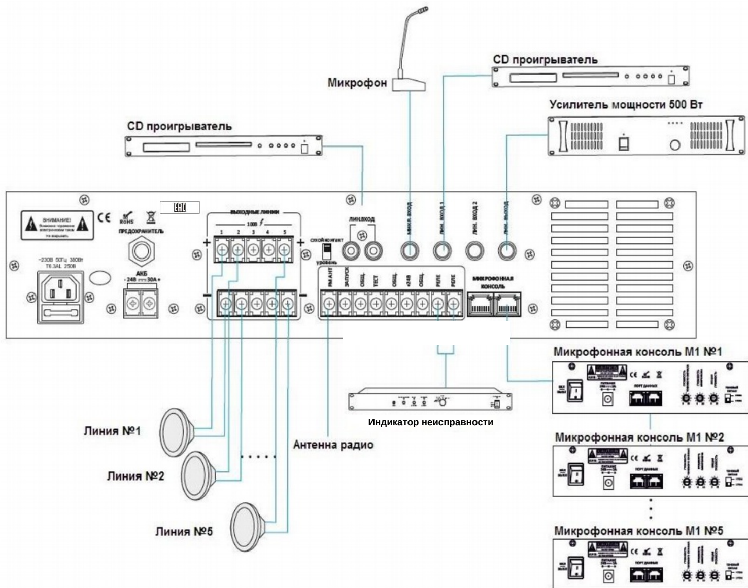
Рис. 2.1. Схема подключения
