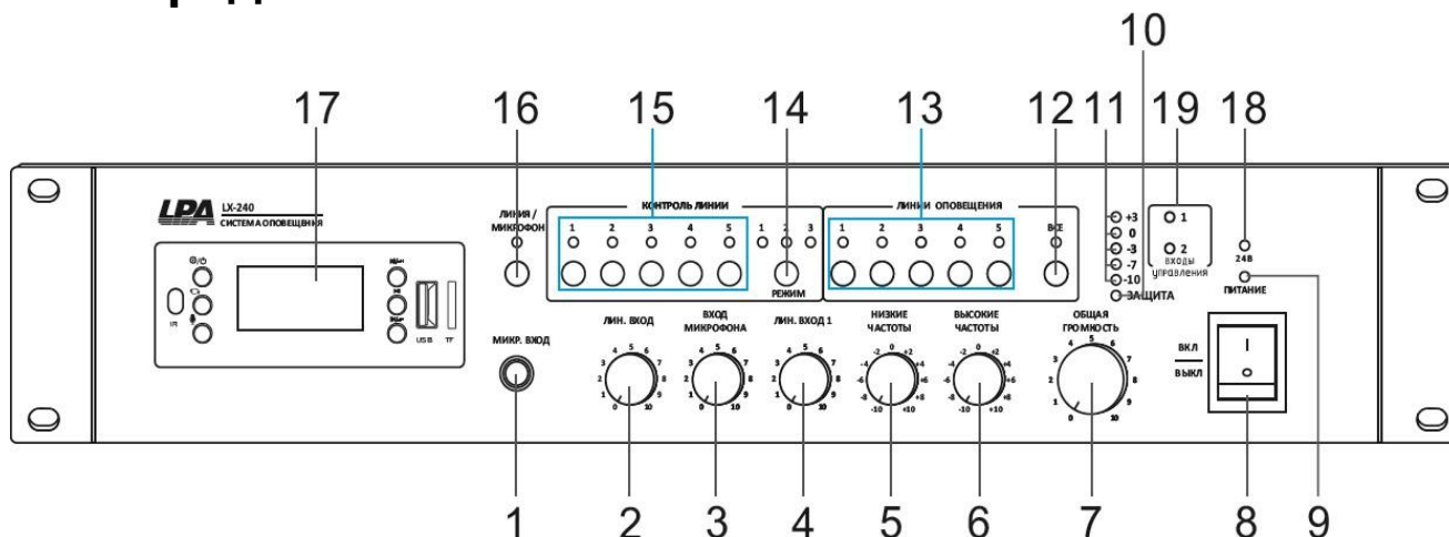
Рис. 1.2. Передняя панель
