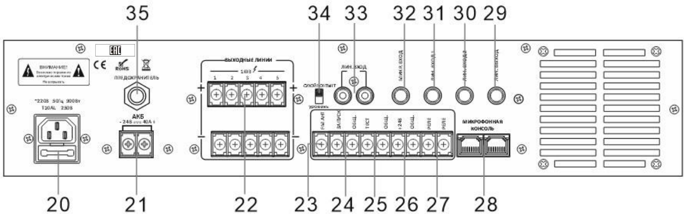
Рис. 1.3. Задняя панель
