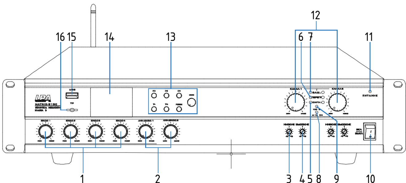
Рис.2.2. передняя панель
