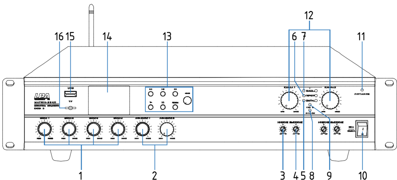
Рис.2.2. передняя панель
