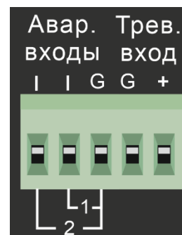
Рис.2.8. Триггерные входы АВАРИЯ и ТРЕВОГА
