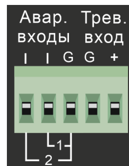
Рис.2.8. Триггерные входы АВАРИЯ и ТРЕВОГА
