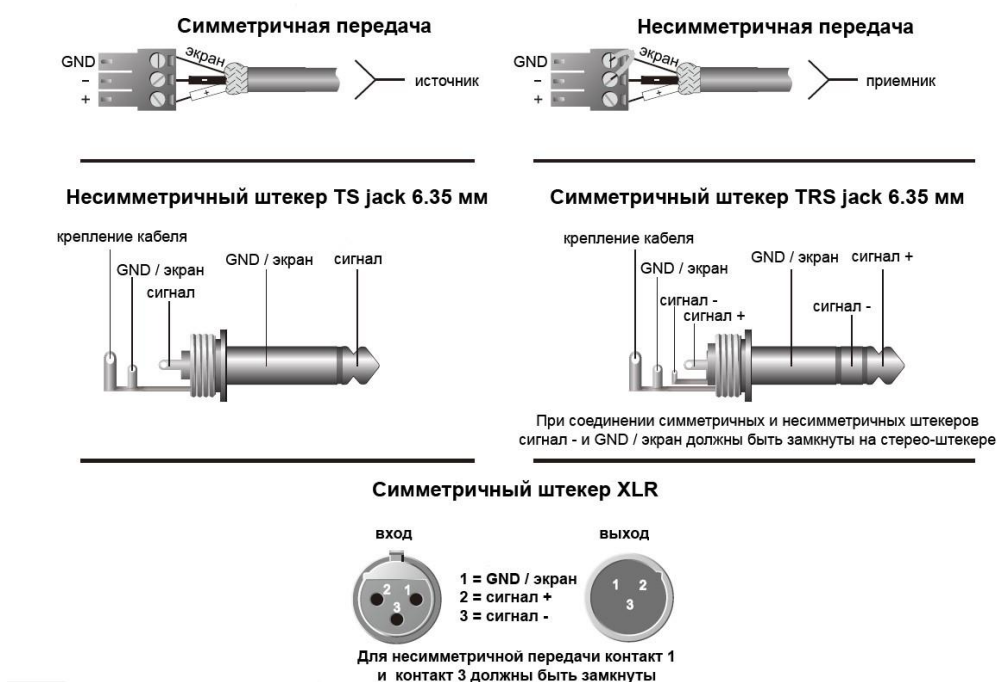
Рис.4.1. Назначение контактов разъемов
