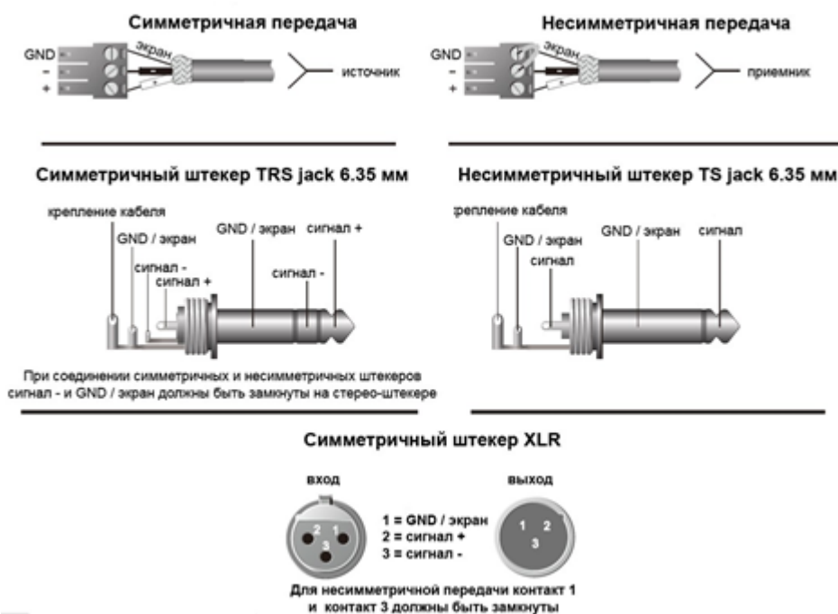
Рис. 4.1 Назначение контактов разъемов
