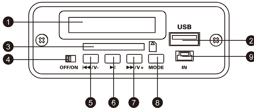
Рис. 3.3. Схема расположения средств управления и разъемов
