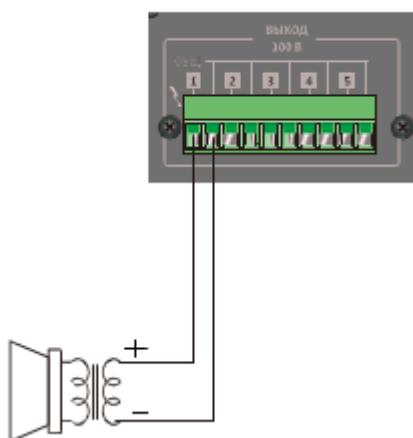
Рис. 2.2. Схема подключения громкоговорителей к LPA-TA-120MZ
