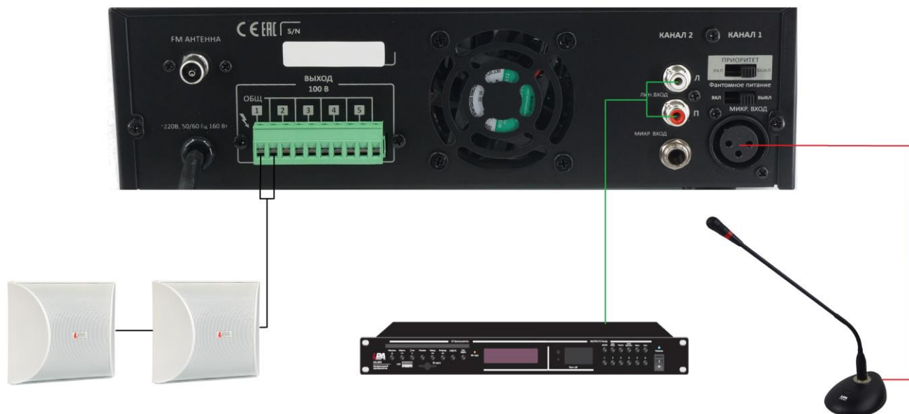
Рис. 2.1 Схема подключения LPA-TA-120MZ
