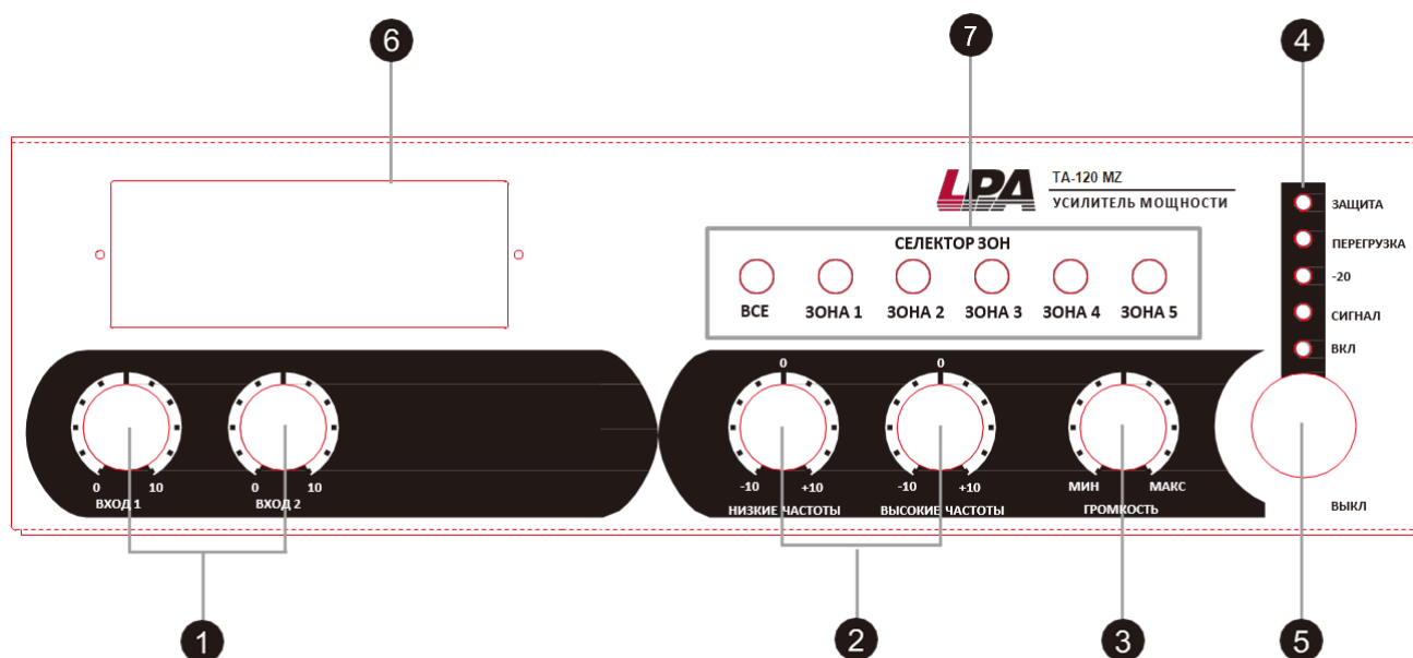
Рис. 3.1. Схема расположения средств управления LPA-TA-120MZ
