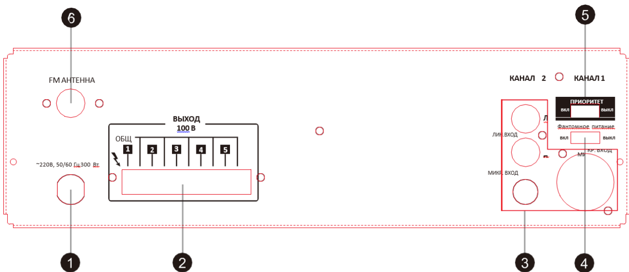
Рис. 3.2. Схема расположения средств управления и разъемов на задней панели
