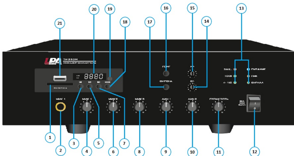
Рис. 3.2. Схема расположения средств управления LPA-TA-350M
