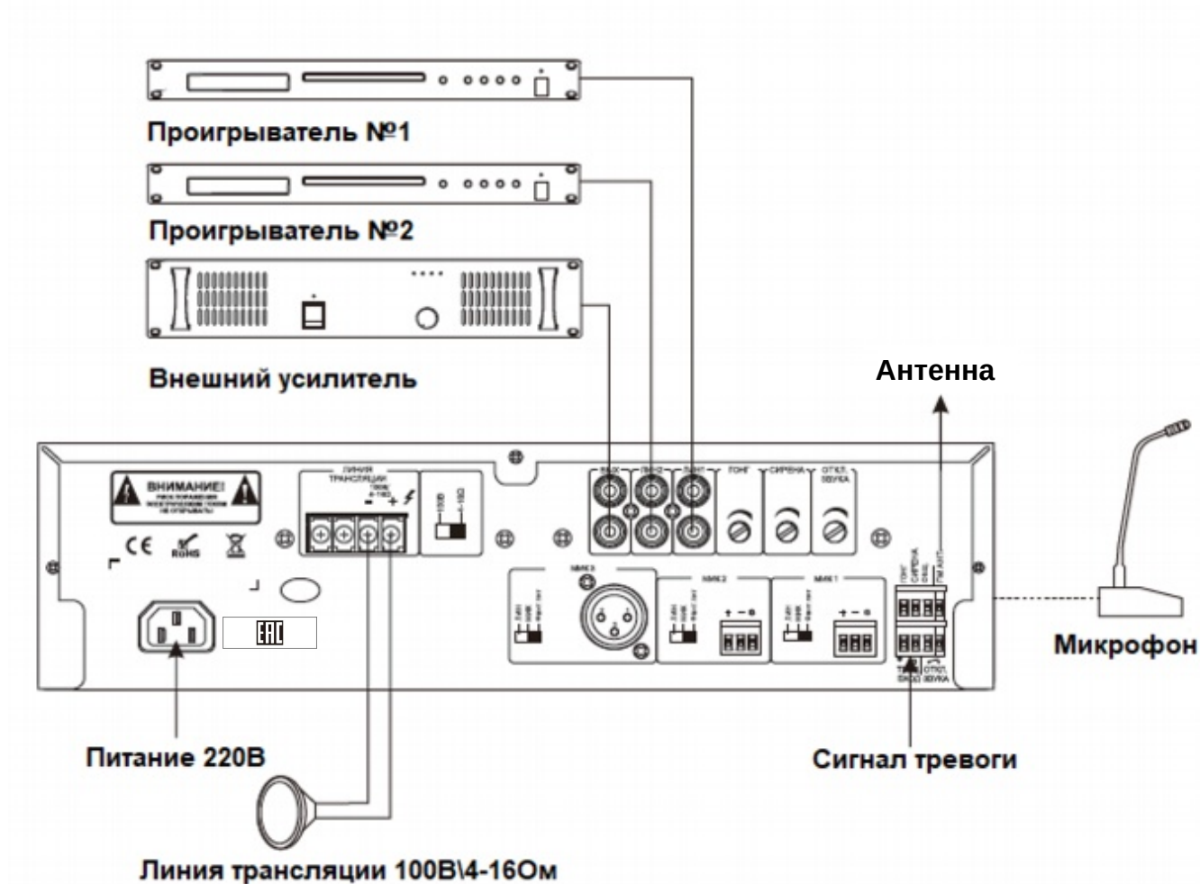
Рис. 2.2. Типовая схема подключения к LPA-TA-350M
