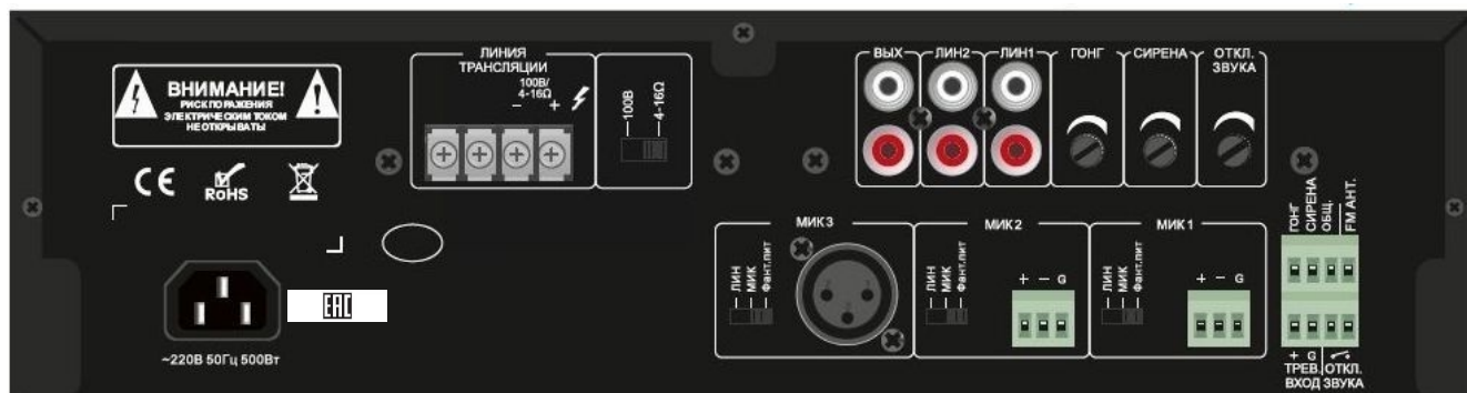
Рис. 2.1. Схема подключения LPA-TA-350M
