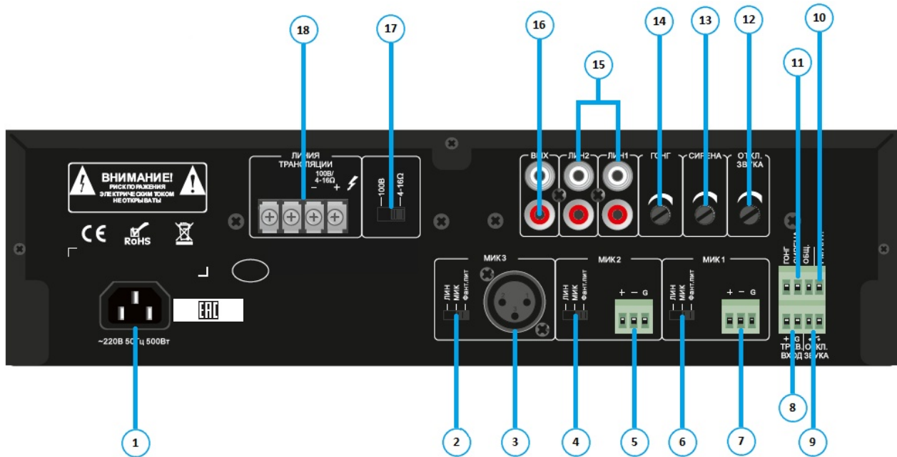
Рис. 3.3. Схема расположения средств управления LPA-TA-350M
