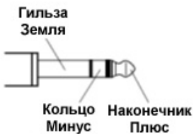
Рис. 4.1. Назначение контактов штекера TRS jack 6.35 мм
