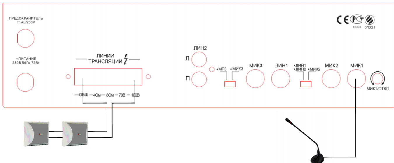
Рис. 2.1. Схема подключения LPA-TA-35KBM
