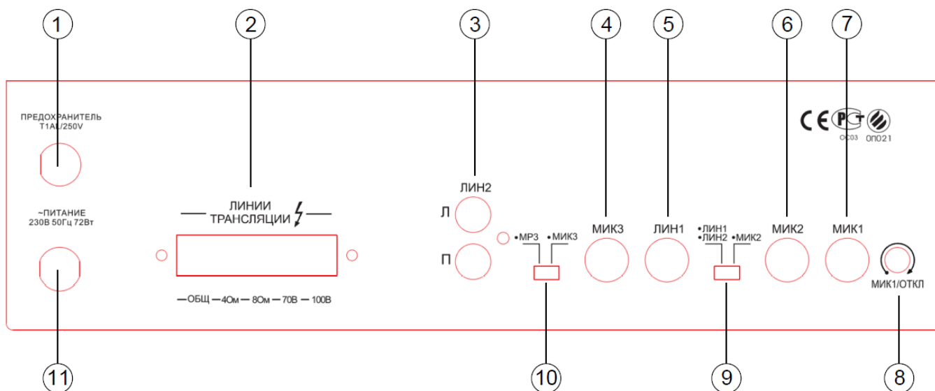
Рис. 3.2. Схема расположения средств управления LPA-TA-35KBM
