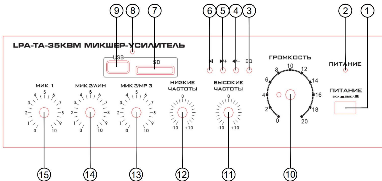
Рис. 3.1. Схема расположения средств управления LPA-TA-35KBM
