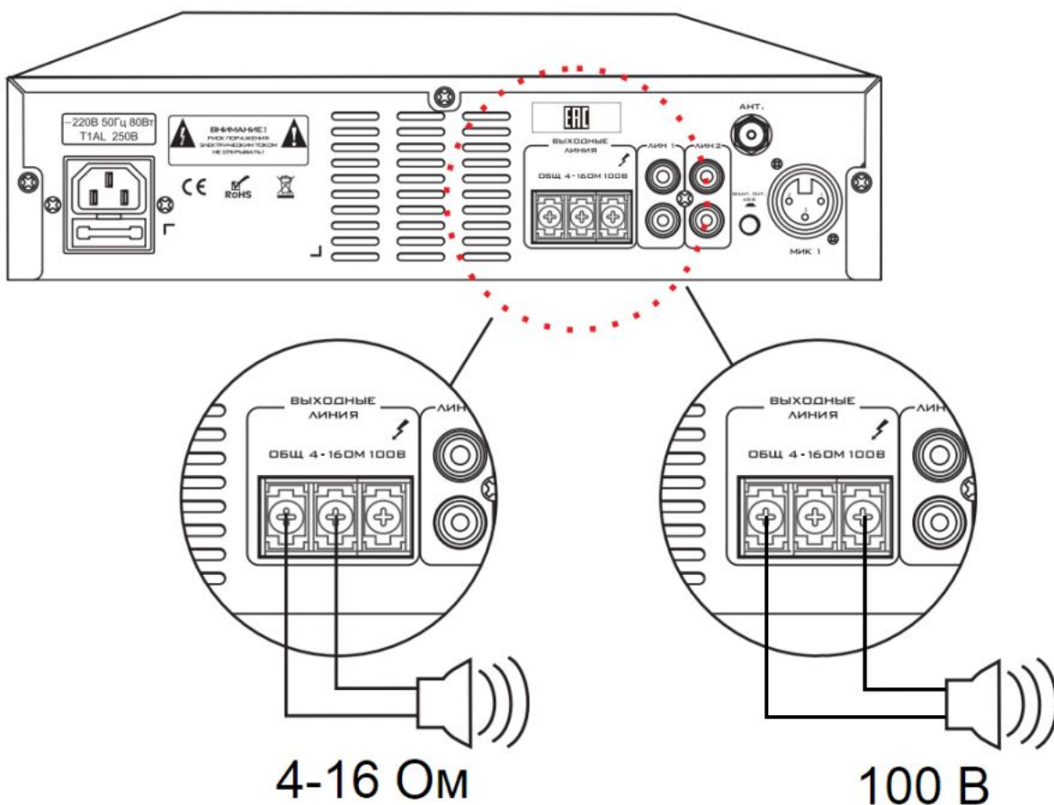
Рис. 2.2. Схема подключения громкоговорителей к LPA-TA-40M
