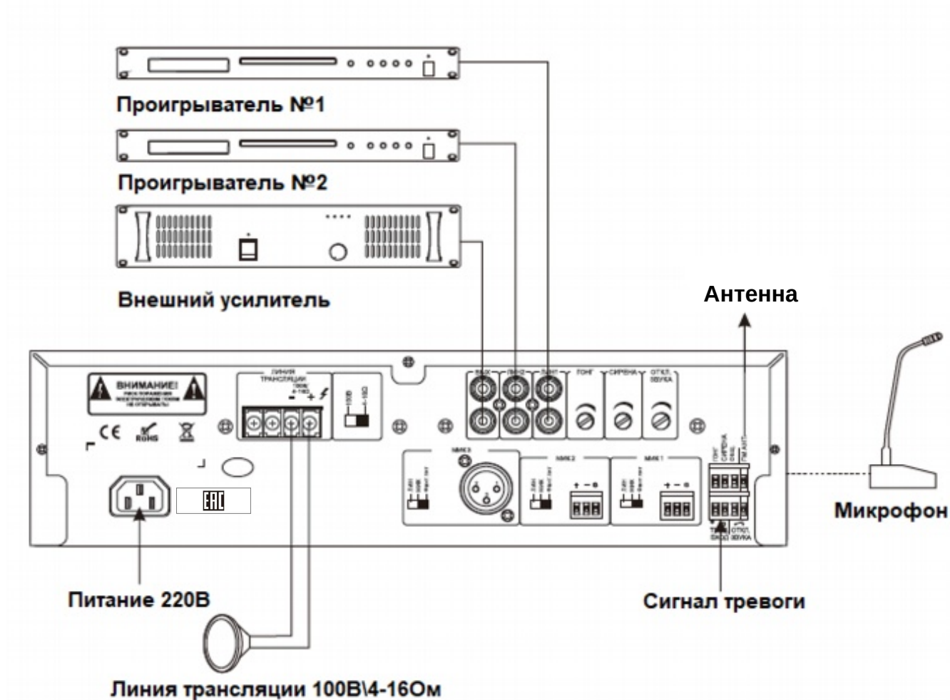
Рис. 2.2. Типовая схема подключения к LPA-TA-500M
