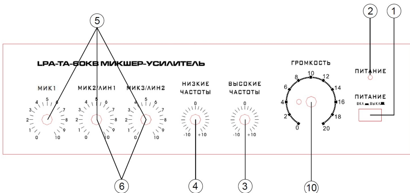
Рис. 3.1. Схема расположения средств управления LPA-TA-60KB
