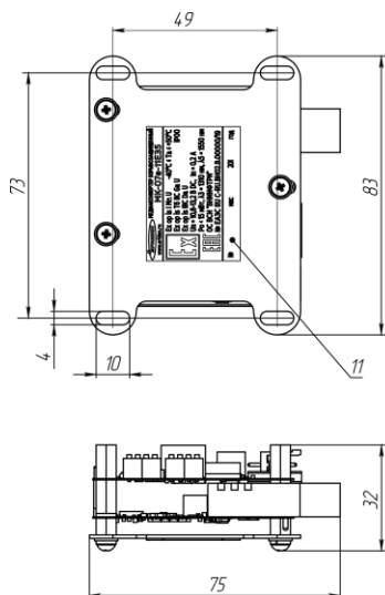
а) размеры без установленной сплайс-кассеты
