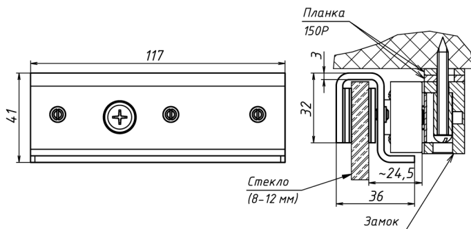
Рисунок 2 - Габаритный чертеж комплекта МК 150-GLU
