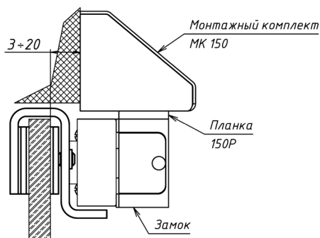
Рисунок 3 – Установка замков ALM-150P и AL-150 Premium на стеклянную дверь с комплектами МК 150 и МК 150-GLU
