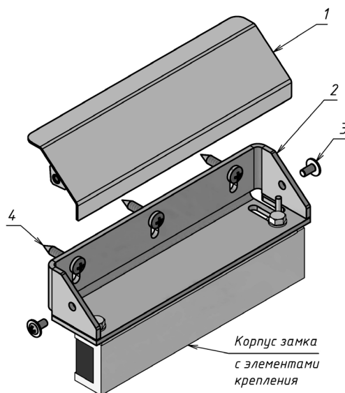
Рисунок 1 – Комплект поставки
