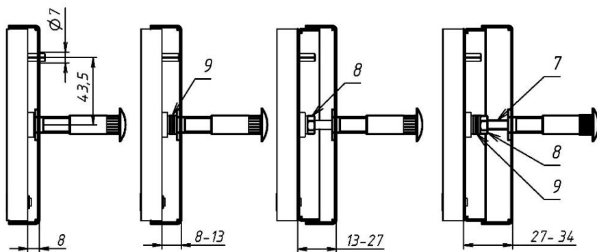
Рисунок 4 – Варианты установки якоря
