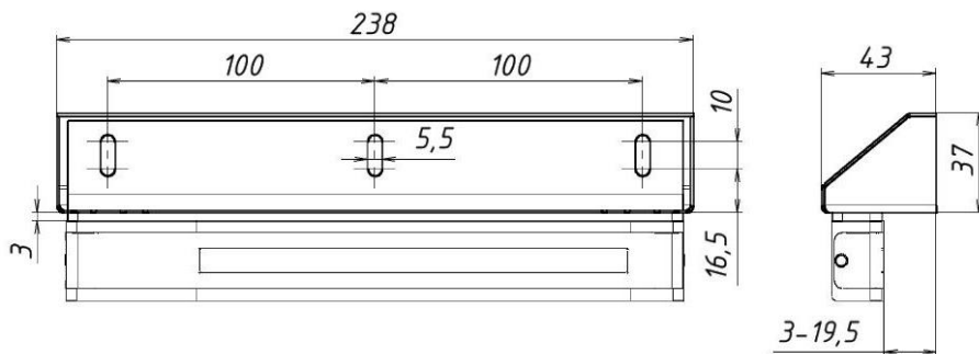
Рисунок 2 – Габаритный чертеж
