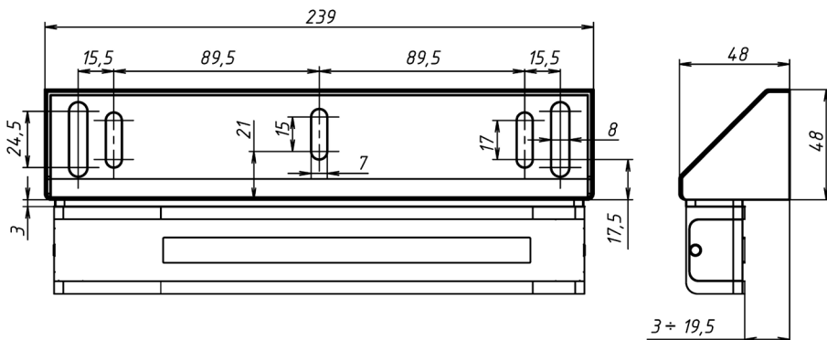
Рисунок 2 – Габаритный чертеж
