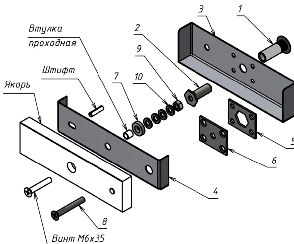
Рисунок 1 – Комплект поставки
