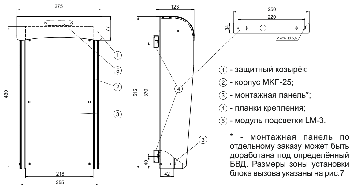
Рис.2 Габаритные и установочные размеры МКФ-25
