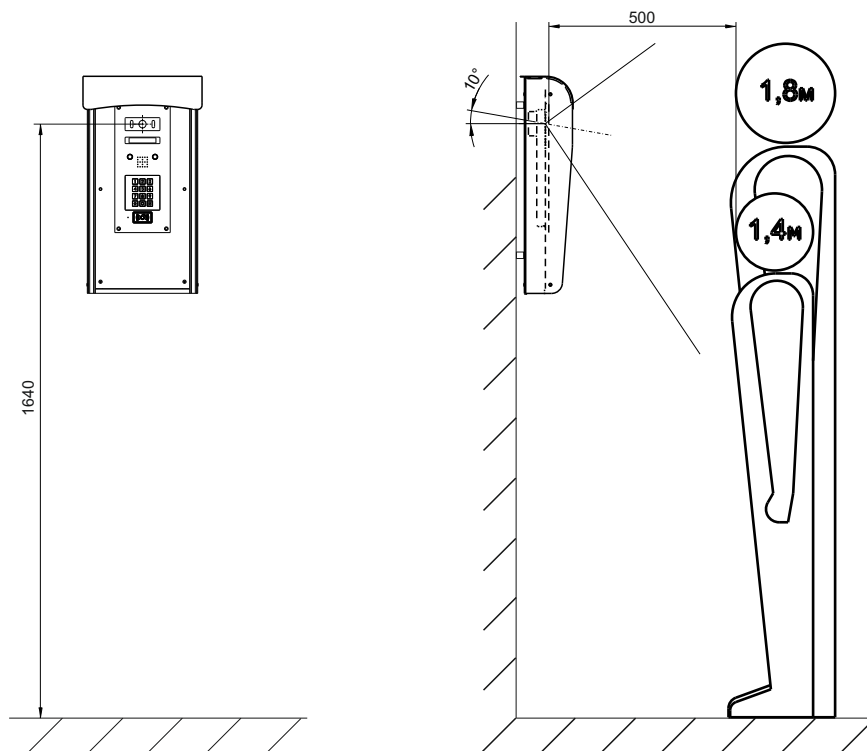
Рис.10 Установлен БВД-440FCB (диагональ объектива телекамеры - 120°)
