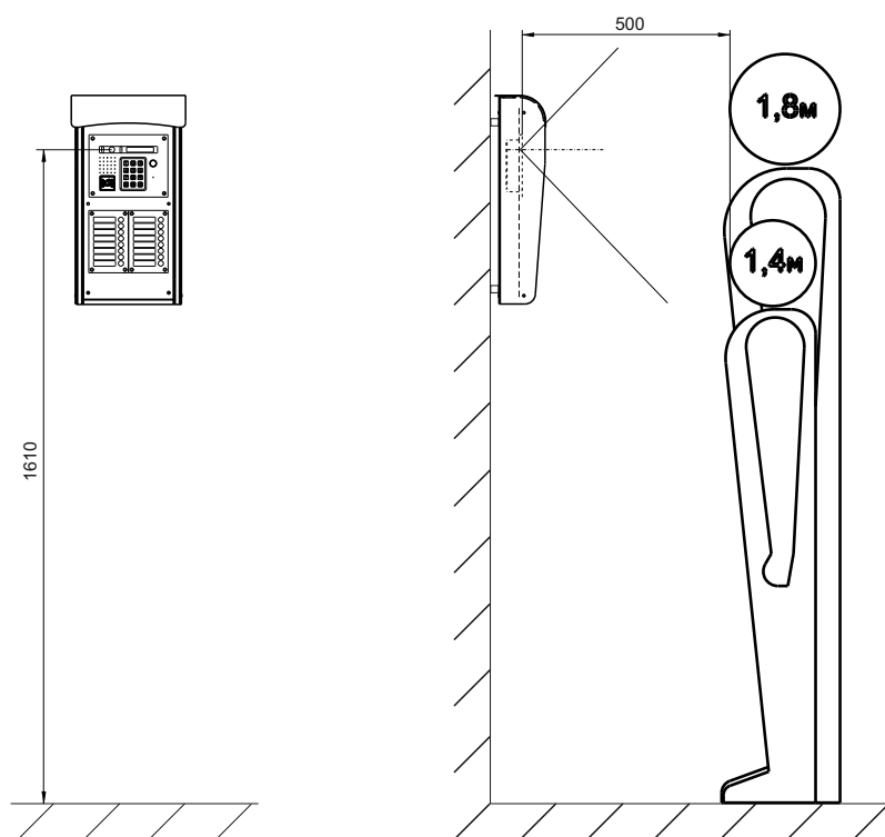
Рис.8 Установлен БВД-432FCB/532FCB (диагональ объектива телекамеры - 120°)
