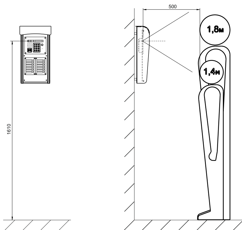
Рис.9 Установлен БВД-533FCBE/733FCBE (диагональ объектива телекамеры - 92°)
