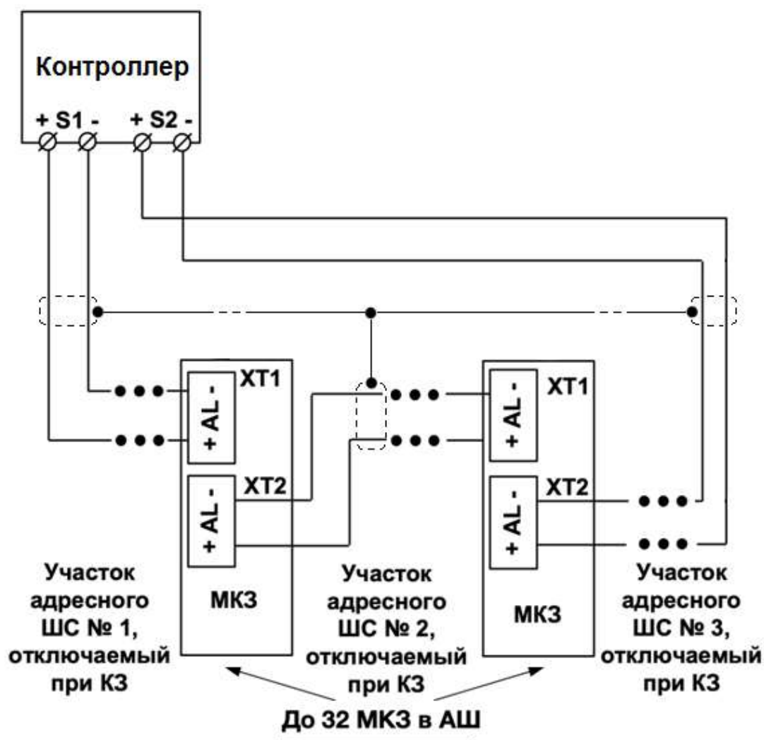
Рис. 2 Подключение МКЗ
