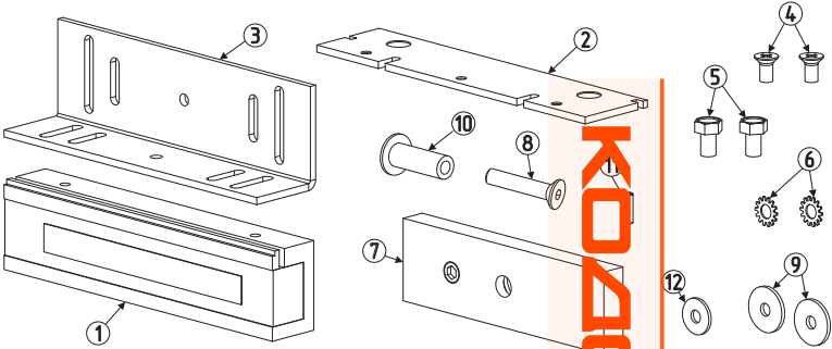
МОНТАЖ ЗАМКА
