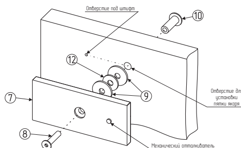
Рисунок 2. Схема установки якоря.
