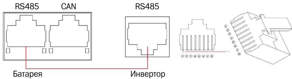
Подключение кабеля обмена данными между батареей и инвертором
