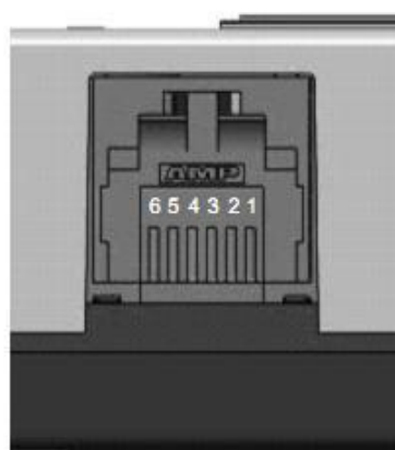
Рисунок 5: 6-контактный разъем Western для электропитания, включения и выключения
