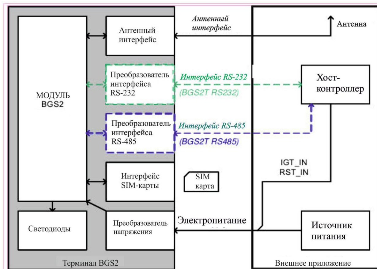
Рисунок 3: Блок-схема
