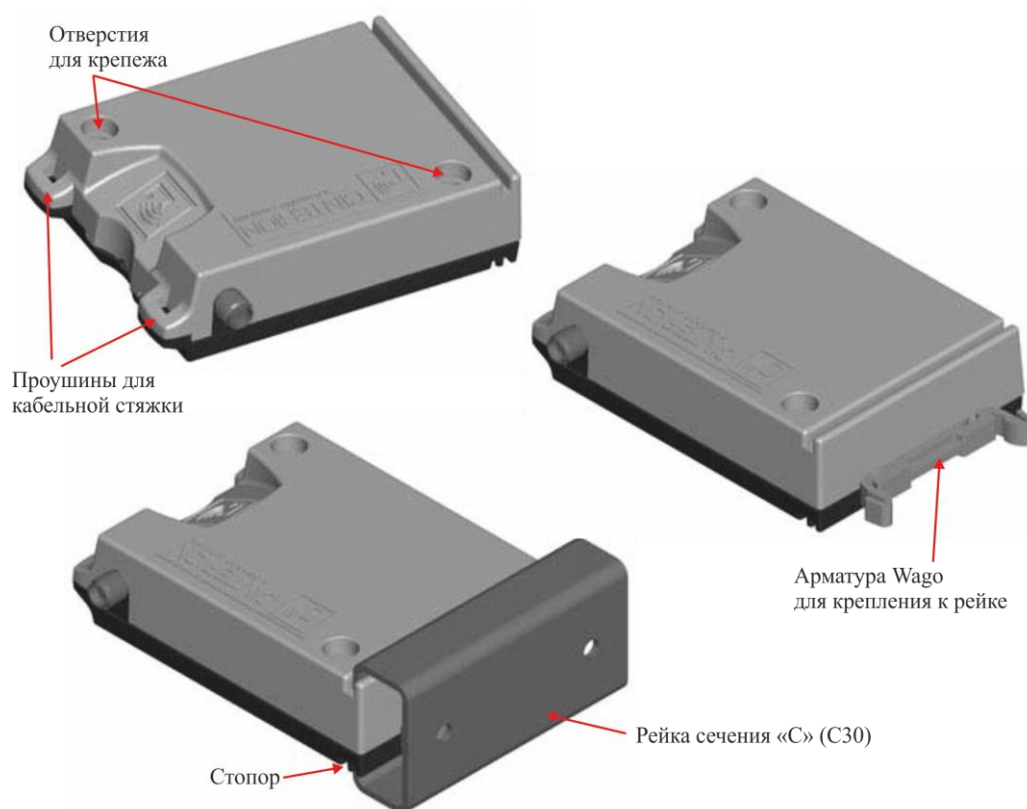
Рисунок 13: Монтаж BGS2T
