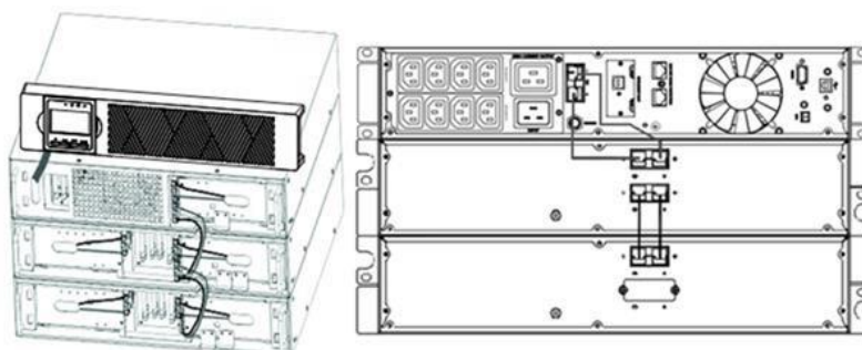
Рисунок 3-4. Подключение разъемов батарейного модуля к ИБП
