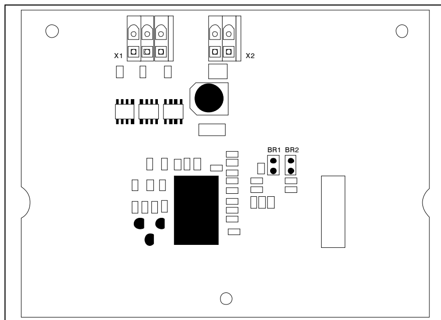
Рис. 5.5: Переключение напряжения вентилятора и клеммной колодки вентилятора на FC-2 или FC-3 на плате цепи управления вентилятора
