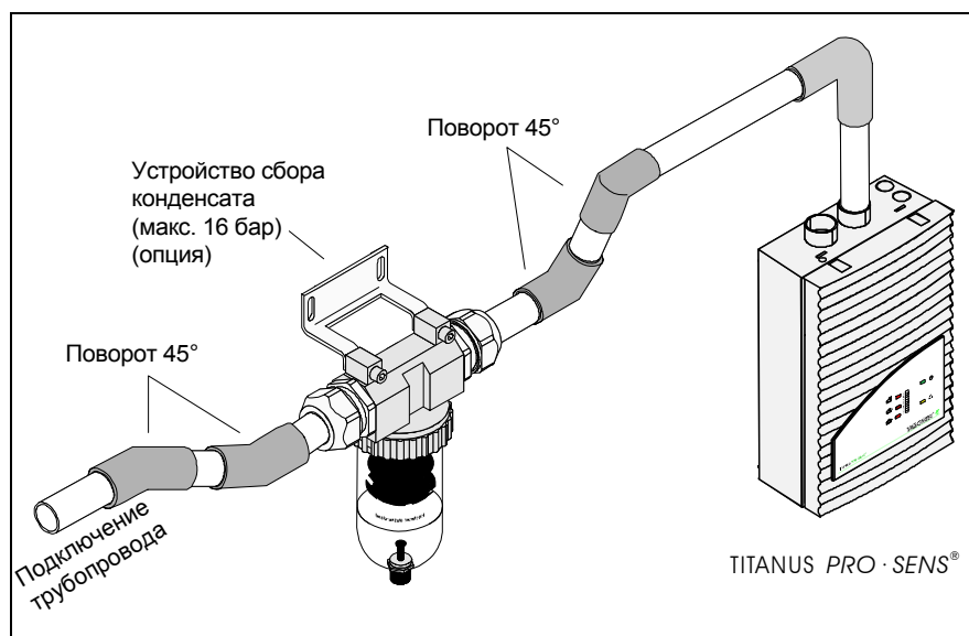
Рис. 2.19: Устройство служит для удаления водяного пара и сбора конденсата из системы труб
