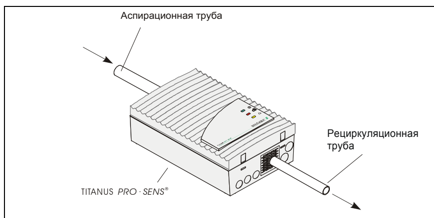
Рис. 2.17: TITANUS PRO·SENS® с рециркуляцией воздуха
