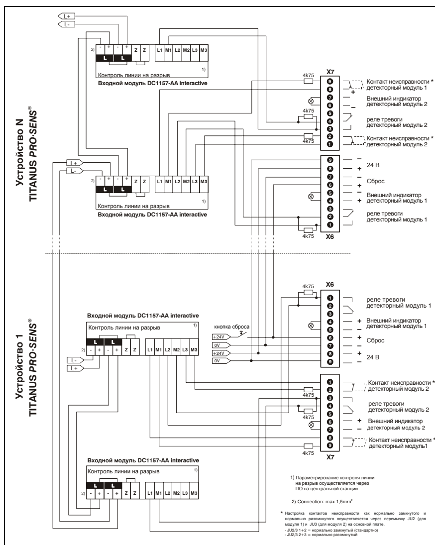
Рис. 5.17: Подключение с применением интерактивной технологии
