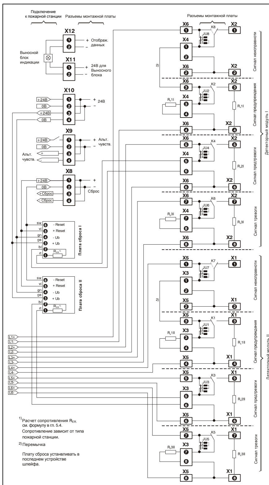
Рис. 5.12: Пример подключения TITANUS® к ПКП с платой сброса
