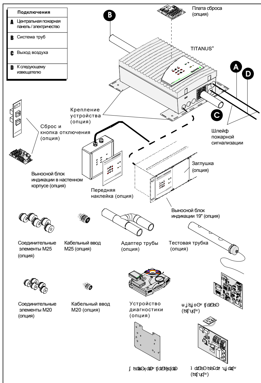
Рис. 2.3: Обзор TITANUS®
