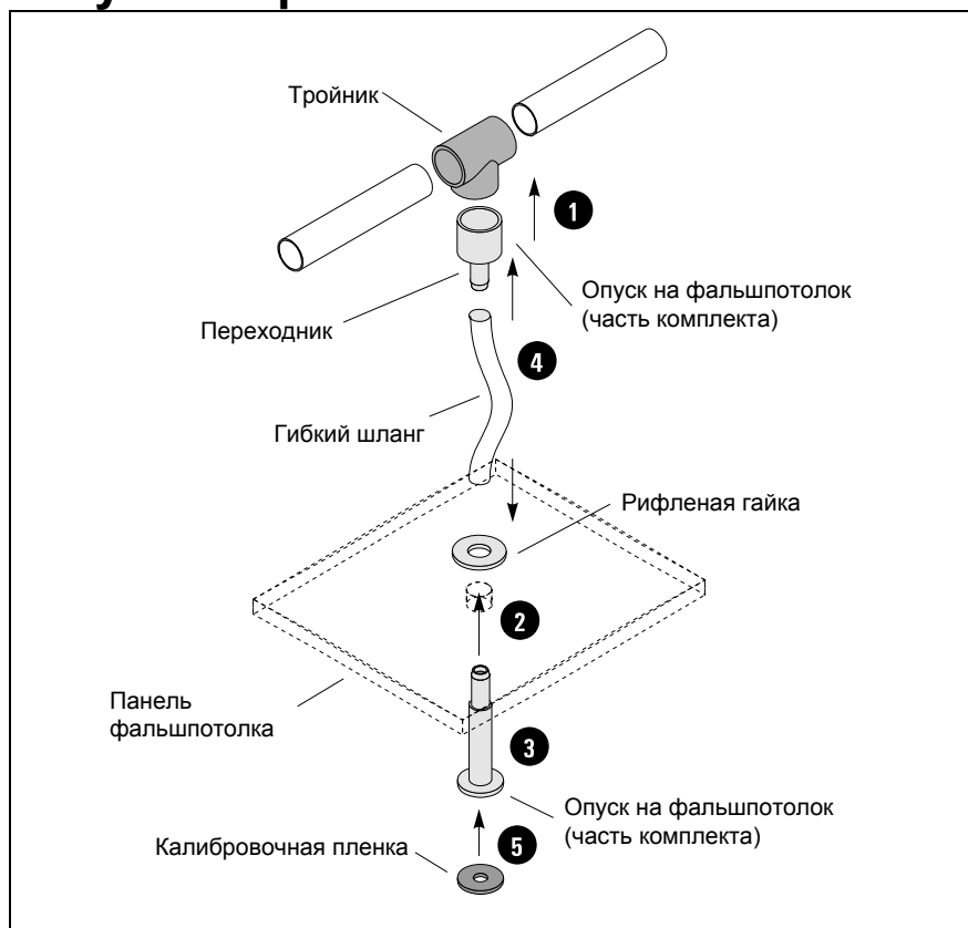
Рис. 6.4 Монтаж опускa на фальшпотолок
